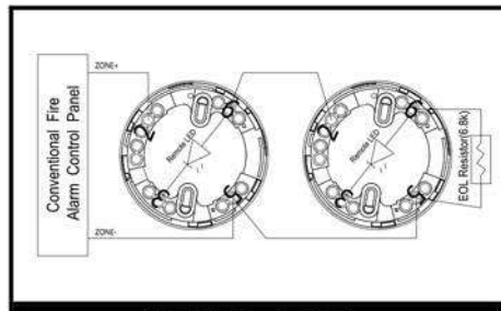
FIGURE1 Terminal Wiring
